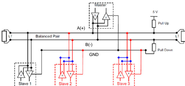
Abbildung 1.4: Beispiele für eine Bus-Kette mit Fail-Safe Terminierung
