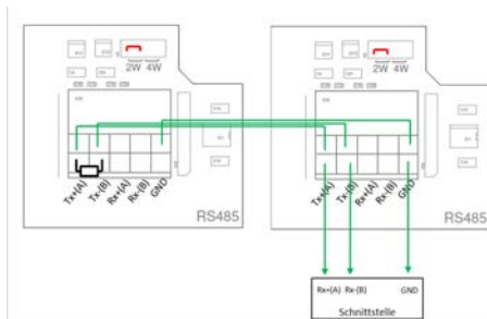
Abbildung 1.3: Beispiele für die Integration eines DUC-MF in eine Bus-Kette mit vernachlässigbarem Rauschen (einfache Terminierung):
