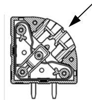
Abbildung 1.2: Detaildarstellung der Push-In Federverbindung (Quelle: www.phoenixcontact.com )
