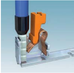
Abbildung 1.1: Push-In Federverbindung (Quelle: www.phoenixcontact.com )
